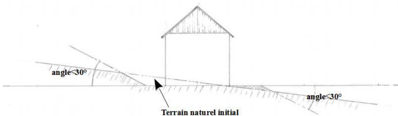
Schéma de principe de calcul de l'angle de pente
